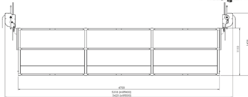
Dimensiones generales Andamio colgante Basic 500 de 2 elevadores
