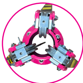
Cabezal con tres poleas
